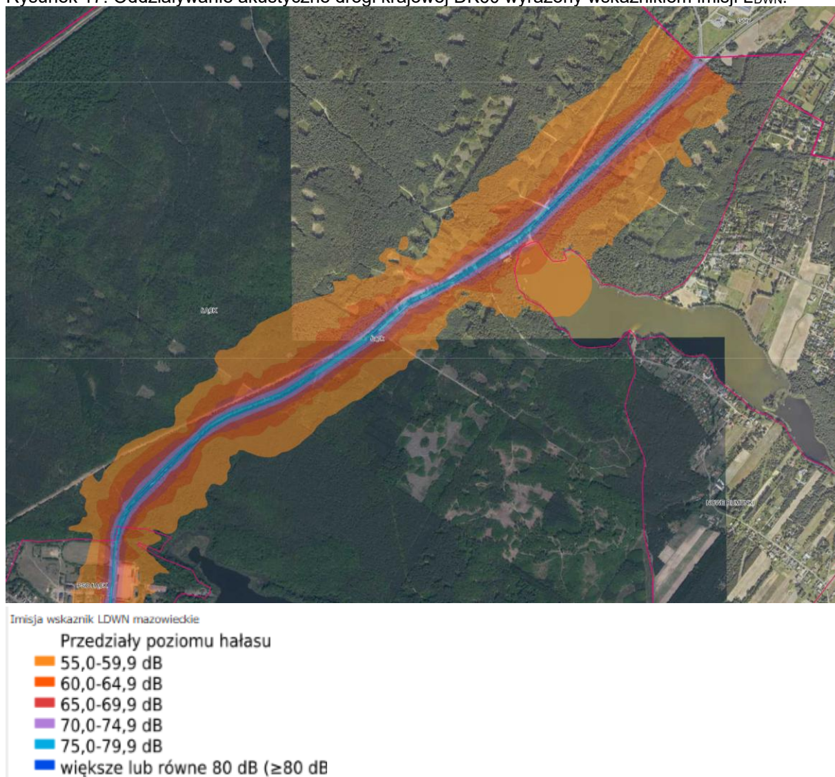
Rysunek 17. Oddziaływanie akustyczne drogi krajowej DK60 wyrażony wskaźnikiem imisji LDWN.
