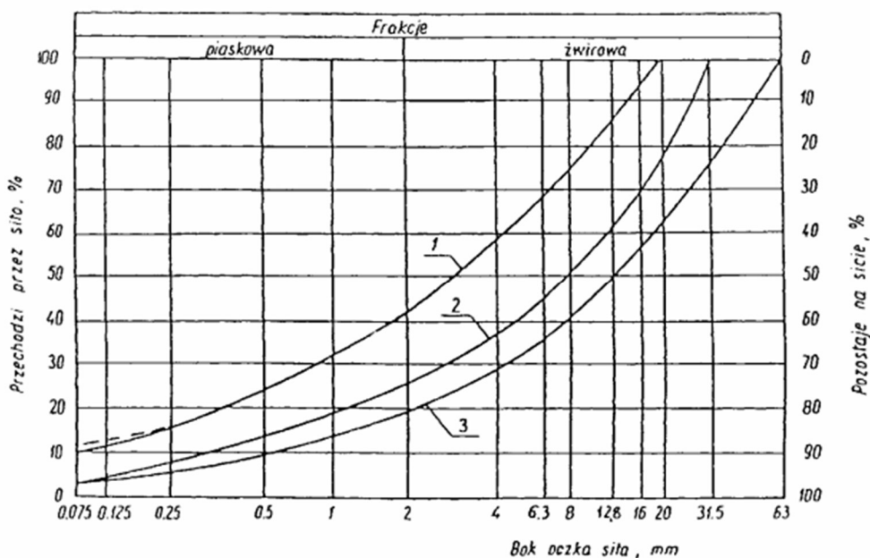
Rysunek 1 Pole dobrego uziarnienia kruszyw na podbudowy wykonane metoda stabilizacji mechanicznej
